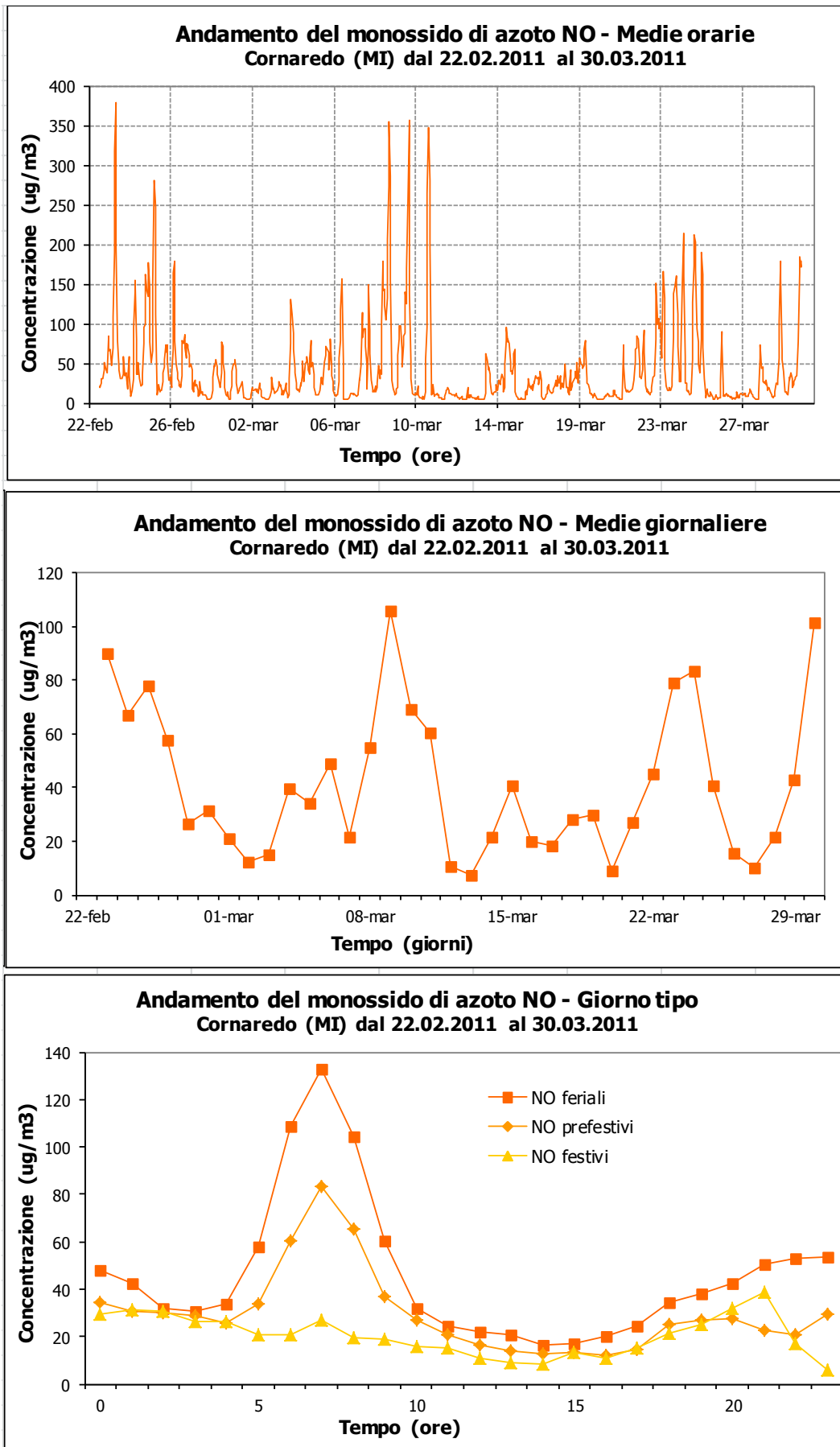
Figura 7: Concentrazioni orarie, medie giornaliere e giorno tipo per NO a Cornaredo nel periodo di misura.
