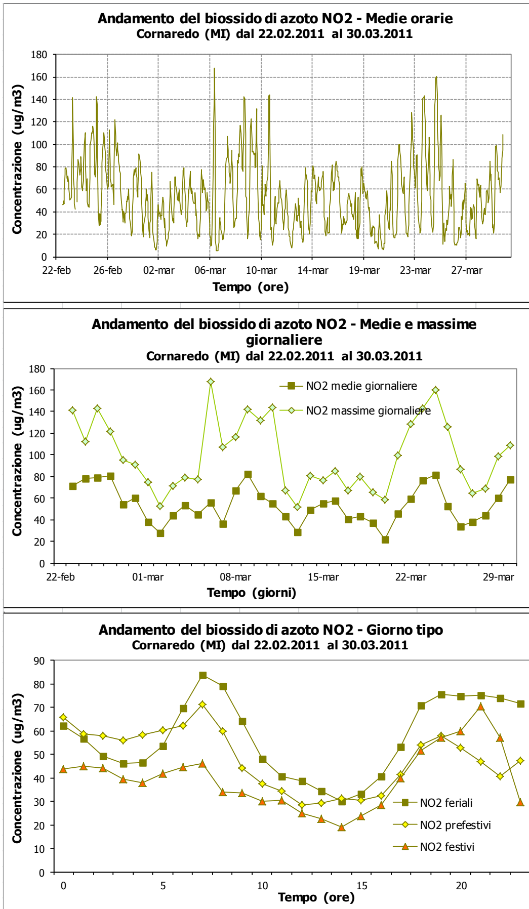
Figura 8: Concentrazioni orarie, medie giornaliere e giorno tipo per NO 2 a Cornaredo nel periodo di misura.
