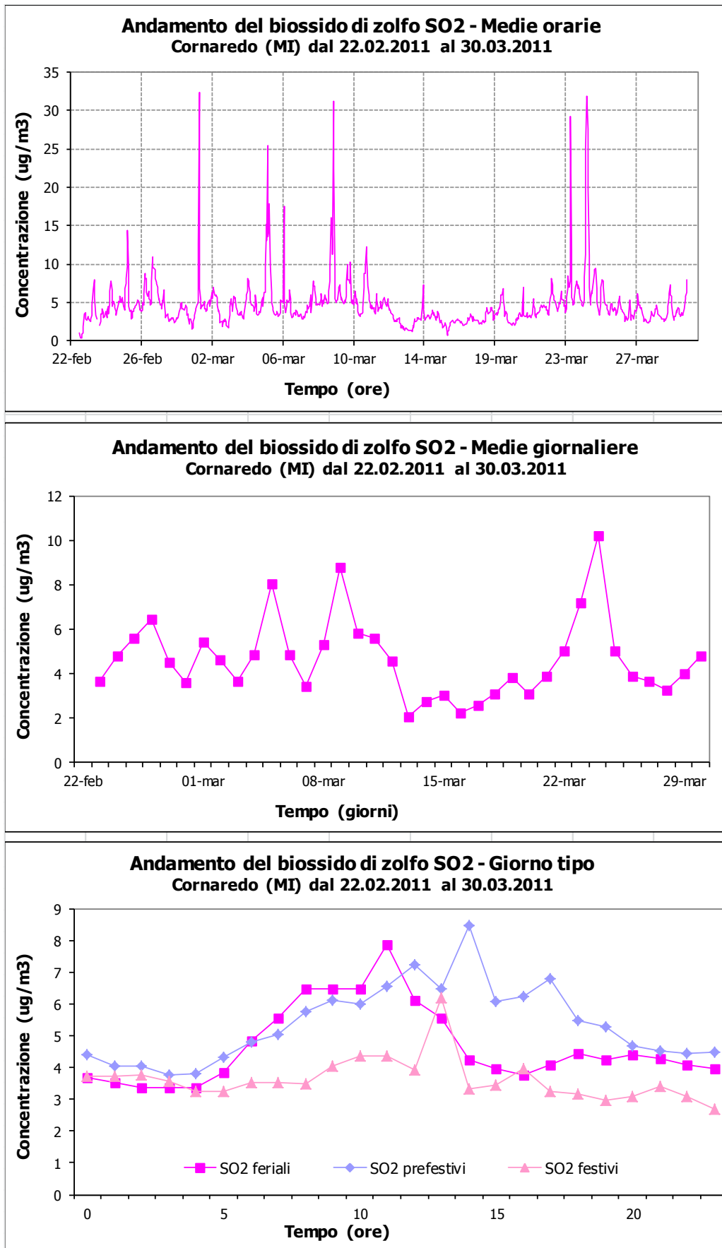
Figura 5: Concentrazioni orarie, medie giornaliere e giorno tipo per SO 2 a Cornaredo nel periodo di misura.
