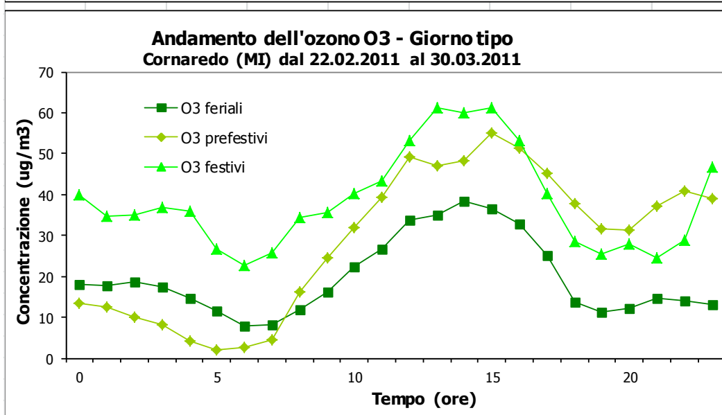
Figura 10: Concentrazioni orarie, medie giornaliere e giorno tipo per O 3 a Cornaredo nel periodo di misura.
