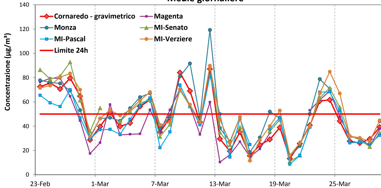
Figura 11: Concentrazioni medie giornaliere di PM10 a Cornaredo e in alcune stazioni della RRQA nel periodo di misura.
