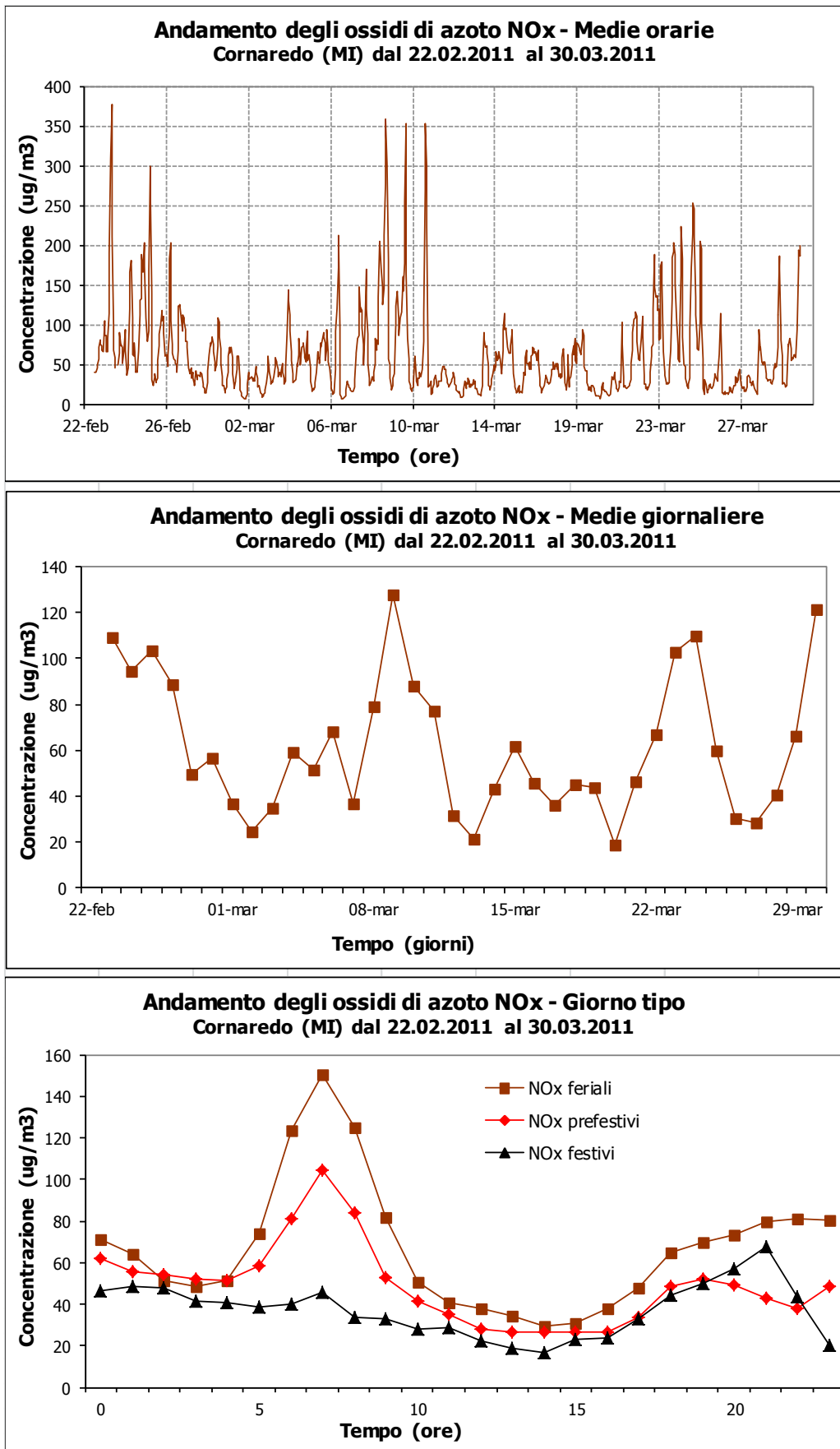
Figura 6: Concentrazioni orarie, medie giornaliere e giorno tipo per NOx a Cornaredo nel periodo di misura.
