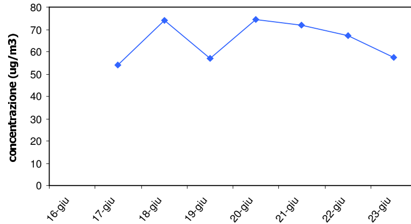
Polveri Totali Sospese-2° periodo Medie Giornaliere
