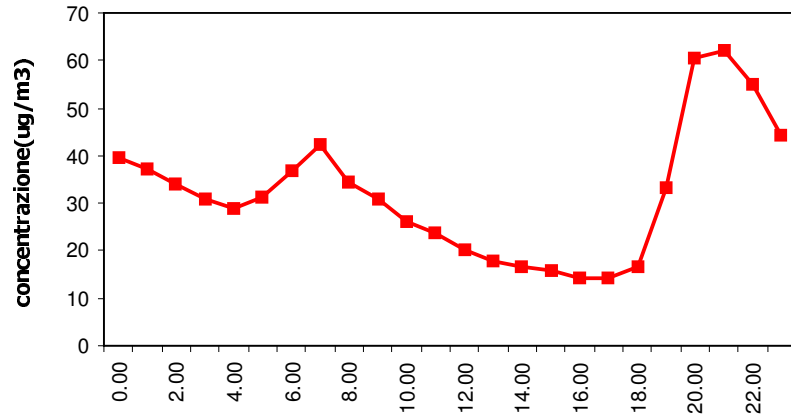
NO2-1° periodo Giorno Tipo
