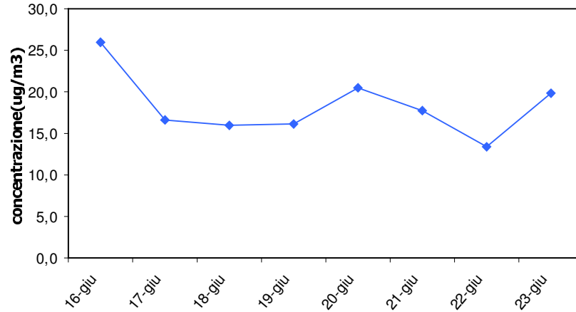
Toluene-2° periodo Medie Giornaliere
