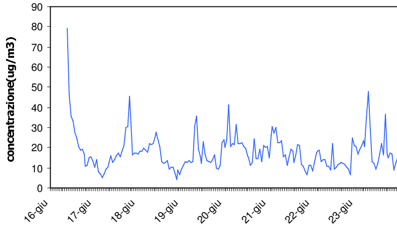
Toluene-2° periodo Concentrazioni Orarie
