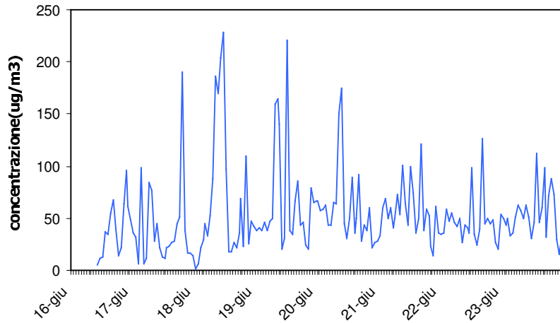
PM-10-2° periodo Concentrazioni Orarie
