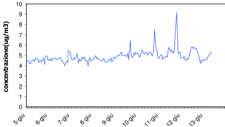
S02-1° periodo Concentrazioni Orarie
