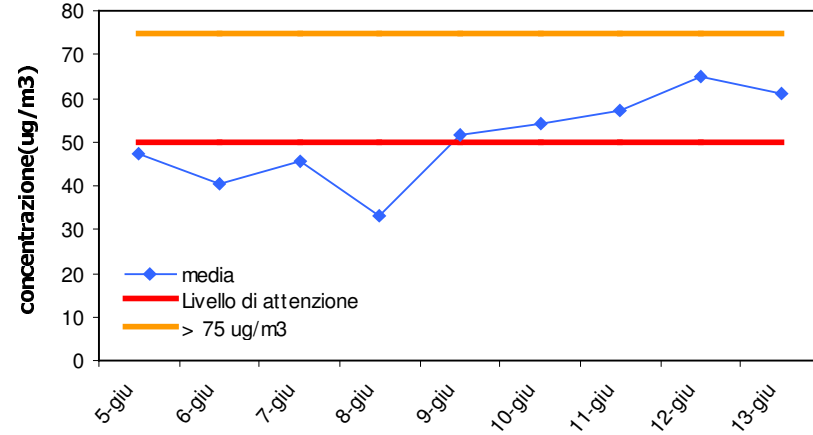
PM-10-1° periodo Medie Giornaliere
