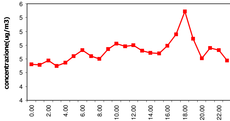
S02-1° periodo Giorno Tipo
