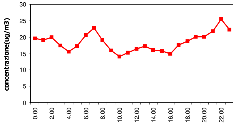
NO2-2° periodo Giorno Tipo
