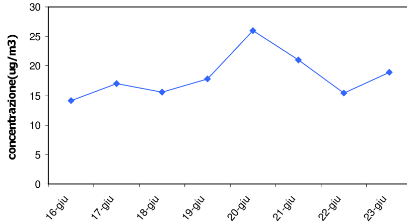
NO2-2° periodo Medie Giornaliere
