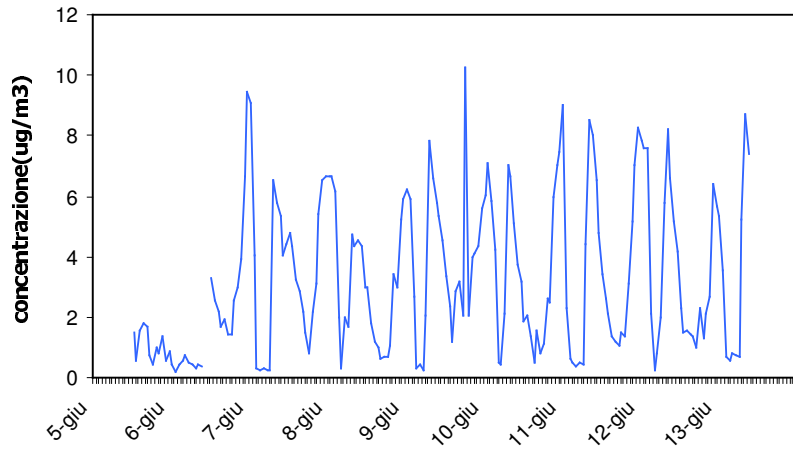
Xilene-1° periodo Concentrazioni Orarie
