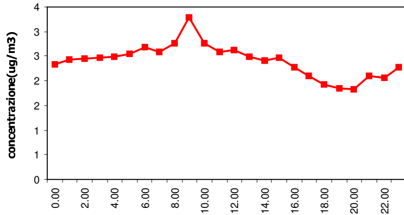
SO2-2° periodo Giorno Tipo
