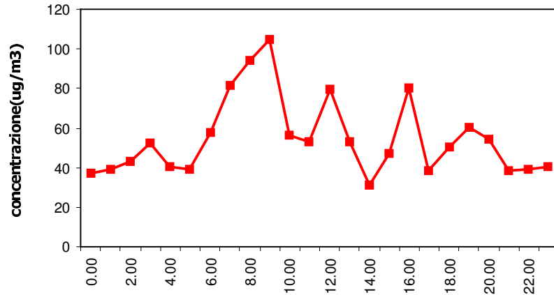
PM-10-2° periodo Giorno Tipo
