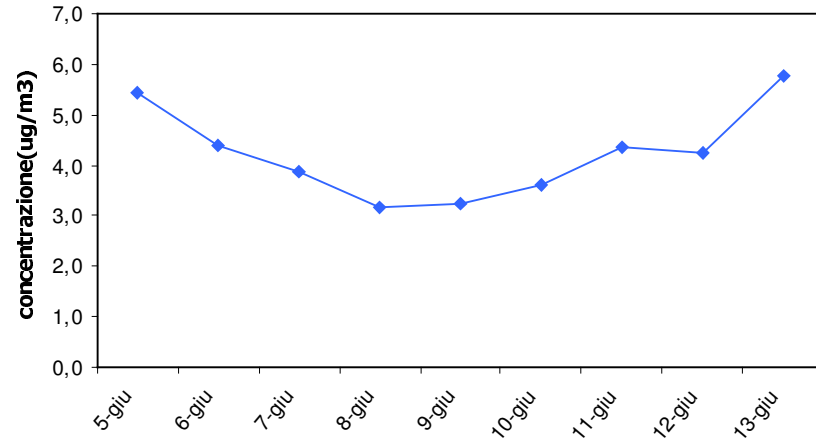
Benzene-1° periodo Medie Giornaliere
