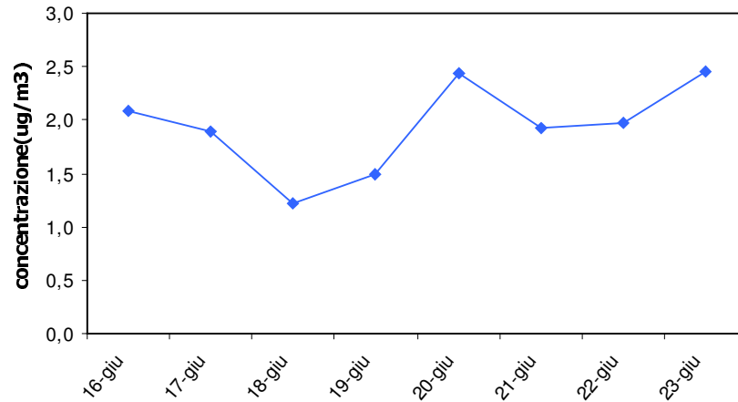
Xilene-2° periodo Medie Giornaliere
