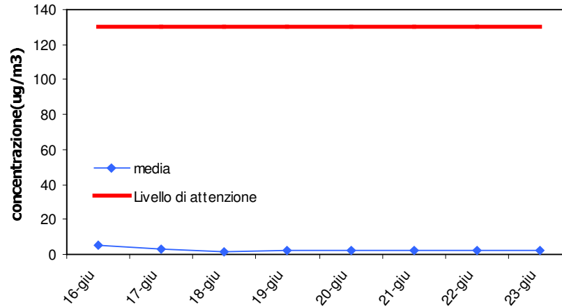
SO2-2° periodo Medie Giornaliere
