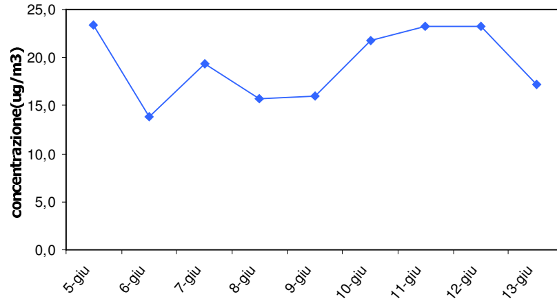
Toluene-1° periodo Medie Giornaliere
