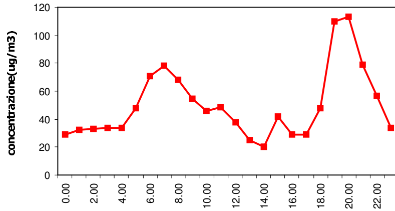
PM-10-1° periodo Giorno Tipo
