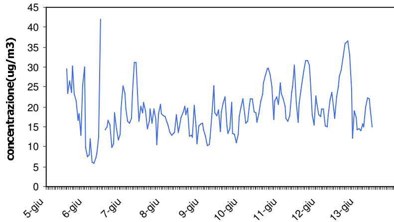
Toluene-1° periodo Concentrazioni Orarie
