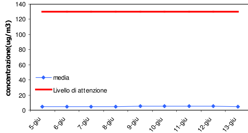
S02-1° periodo Medie Giornaliere
