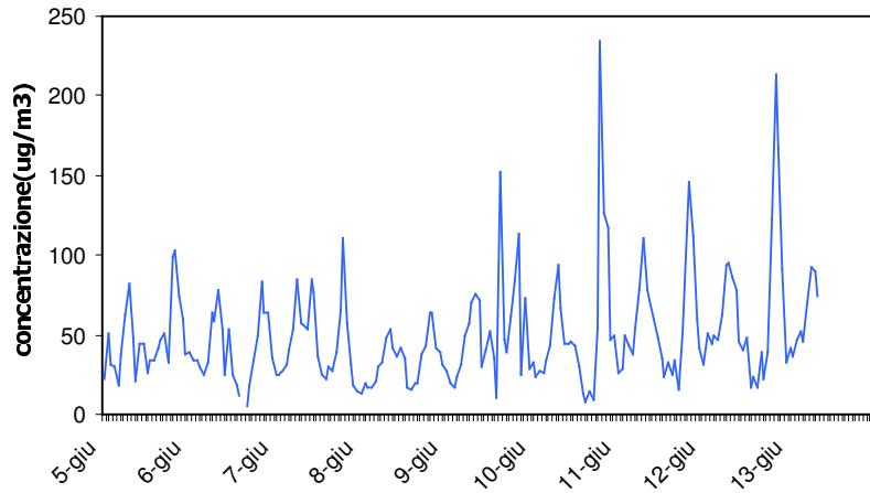
PM-10-1° periodo Concentrazioni Orarie
