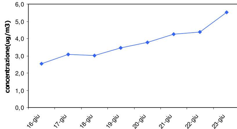
Benzene-2° periodo Medie Giornaliere
