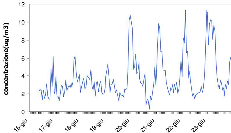
Benzene-2° periodo Concentrazioni Orarie
