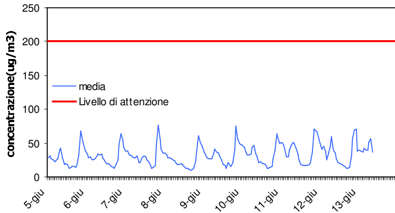
NO2-1° periodo Giorno Tipo
