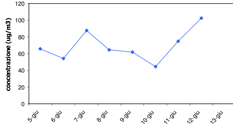
Polveri Totali Sospese-1° periodo Medie Giornaliere
