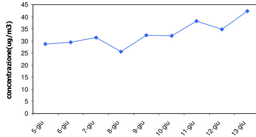
NO2-1° periodo Medie Giornaliere
