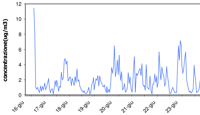
Xilene-2° periodo Concentrazioni Orarie
