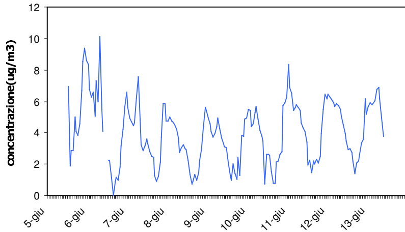
Benzene-1° periodo Concentrazioni Orarie
