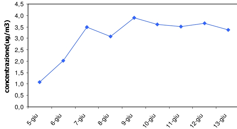
Xilene-1° periodo Medie Giornaliere
