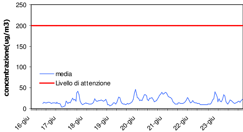
NO2-2° periodo Giorno Tipo
