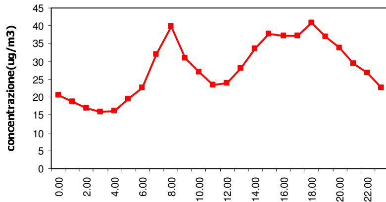
PM-10 Giorno Tipo
