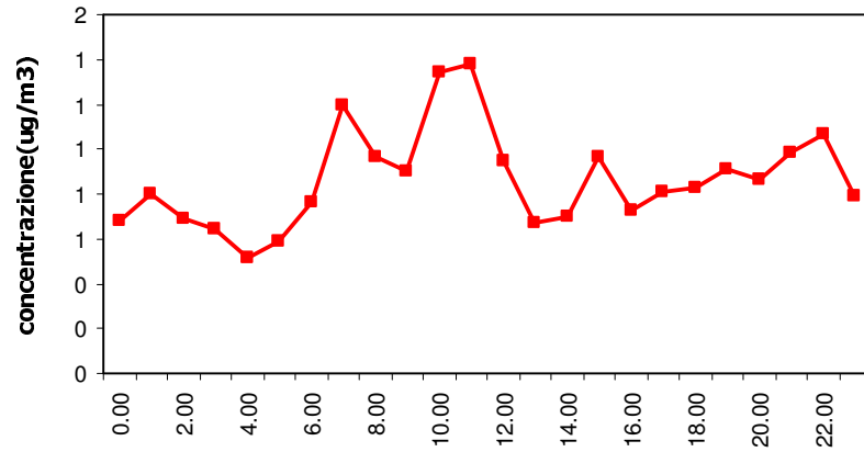
Xilene Giorno Tipo
