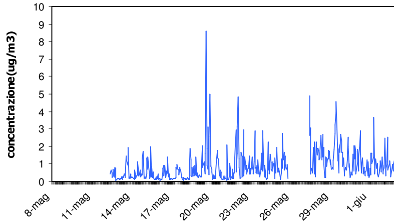
Xilene Concentrazioni Orarie
