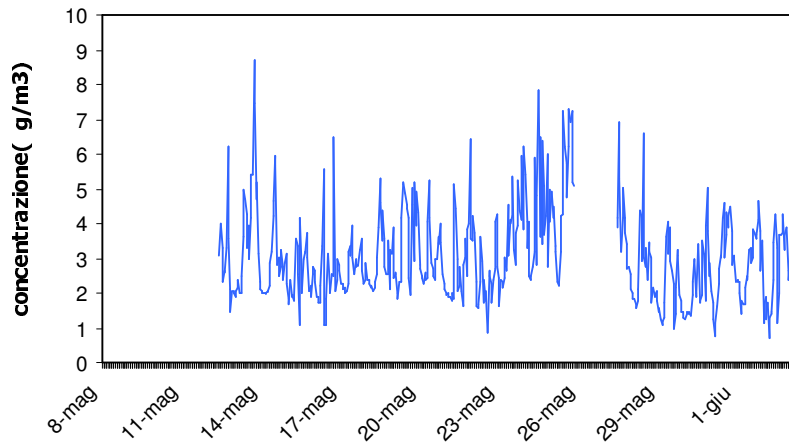
Benzene Concentrazioni Orarie
