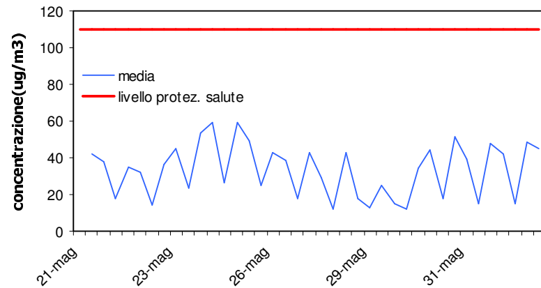
Ozono Concentrazioni Media 8 ore
