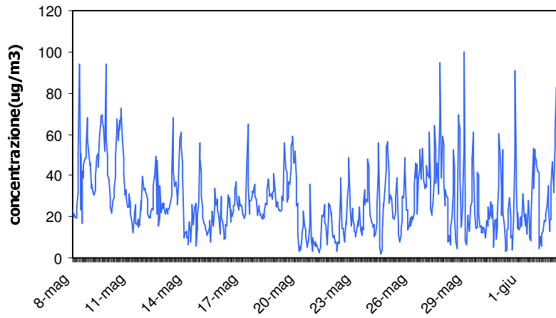
PM-10 Concentrazioni Orarie
