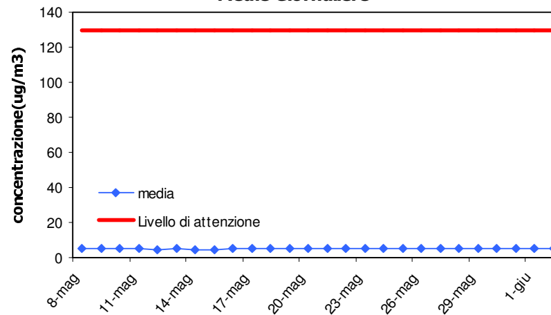
SO2 Medie Giornaliere
