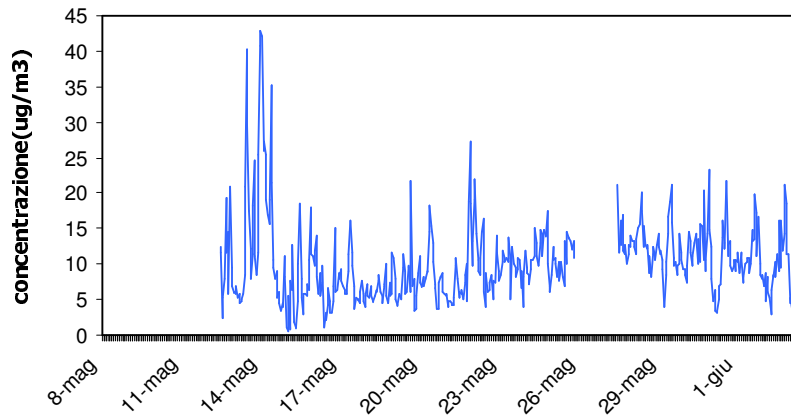
Toluene Concentrazioni Orarie
