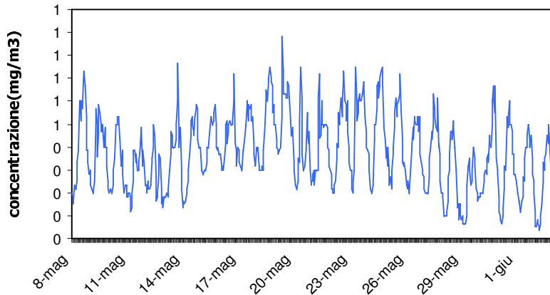
CO Giorno Tipo
