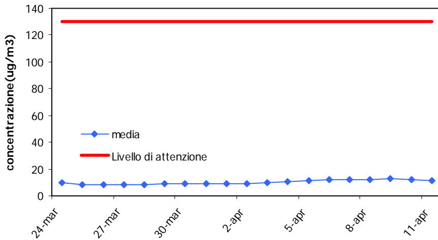
SO2 - Postazione 1 Medie Giornaliere
