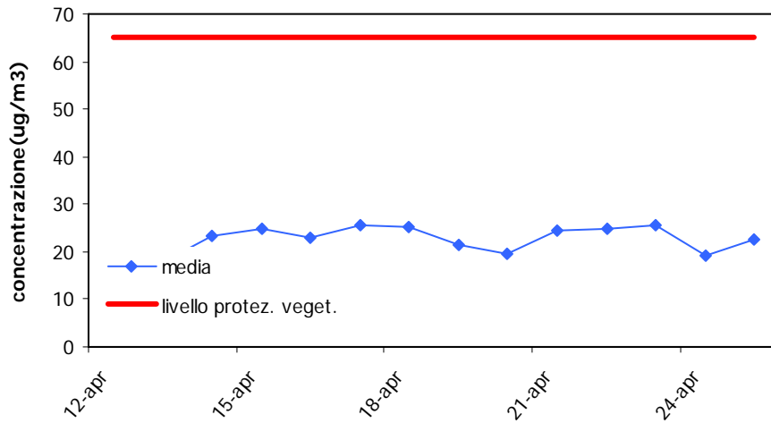
Ozono - Postazione 2 Medie Giornaliere
