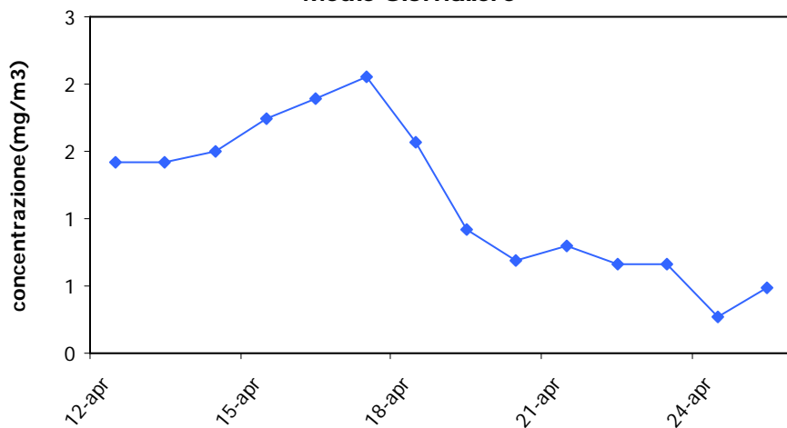
CO - Postazione 2 Medie Giornaliere
