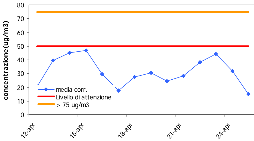
PM-10 - Postazione 2 Medie Giornaliere
