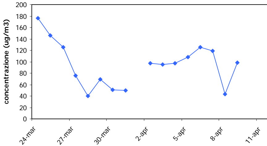
Polveri Totali Sospese - Postazione 1 Medie Giornaliere
