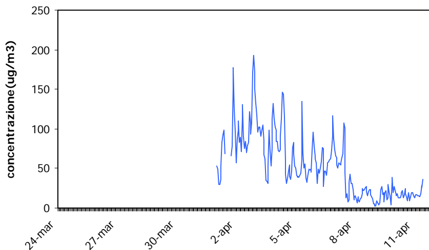
PM-10 - Postazione 1 Concentrazioni Orarie
