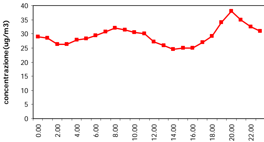
NO2 - Postazione 1 Giorno Tipo
