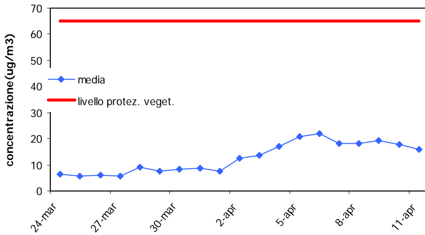
Ozono - Postazione 1 Medie Giornaliere
