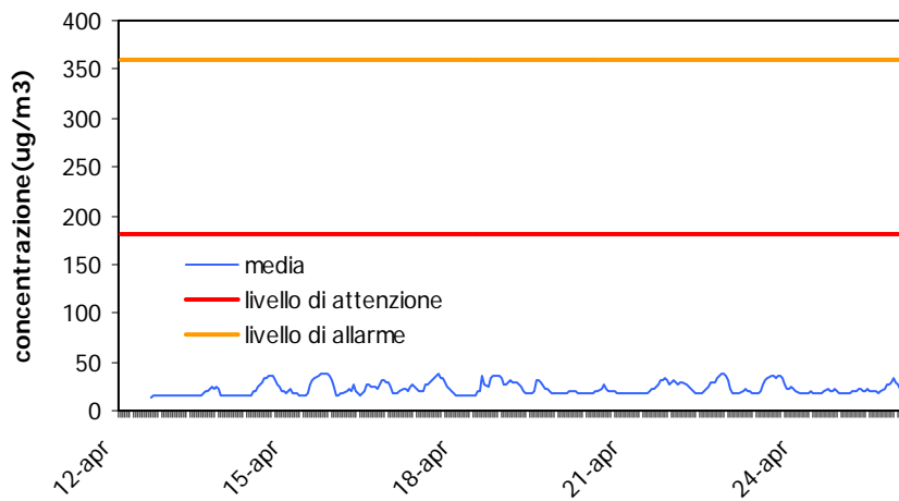
Ozono - Postazione 2 Concentrazioni Orarie
