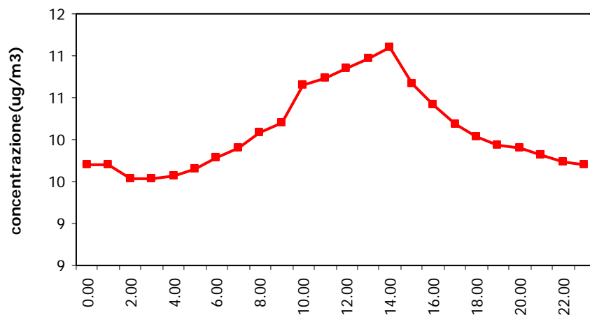
SO2 - Postazione 1 Giorno Tipo
