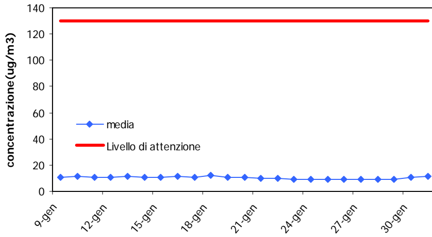
S02 Medie Giornaliere
