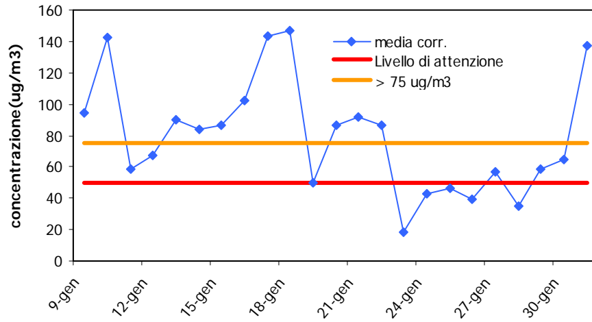
PM-10 Medie Giornaliere
