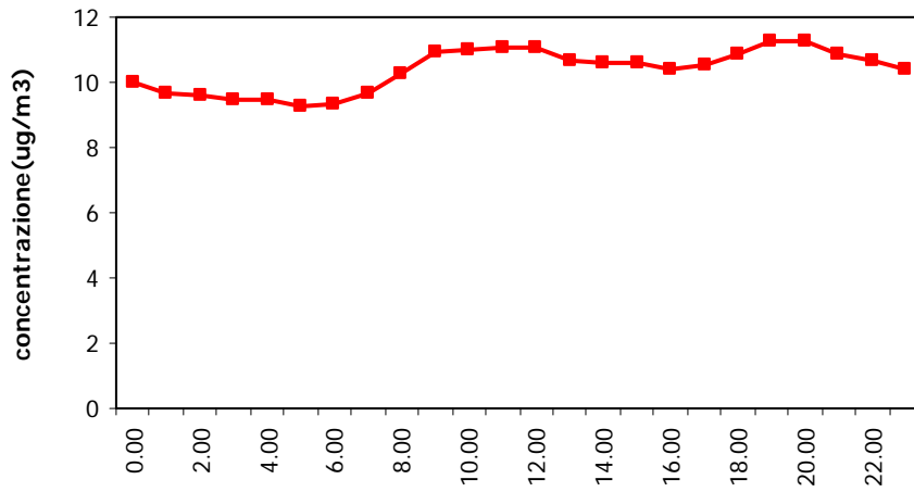
S02 Giorno Tipo
