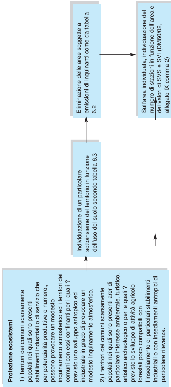
Figura n. A.2: Protezione agli ecosistemi. Individuazione aree idonee
