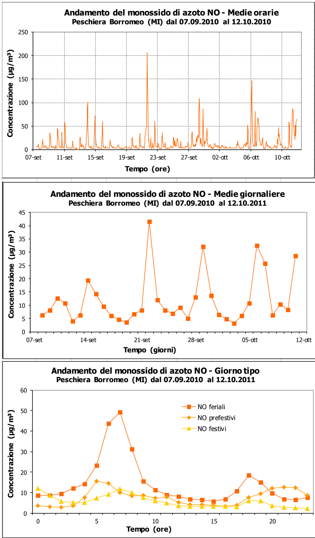
Figura 7: Concentrazioni orarie, medie giornaliere e giorno tipo per NO a Peschiera Borromeo nel periodo di misura.
