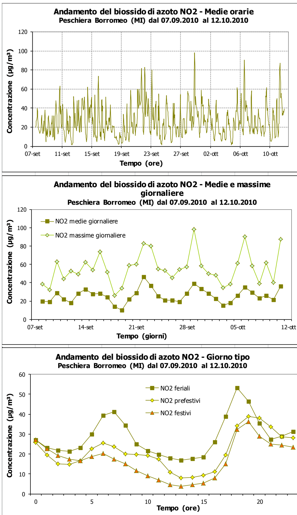
Figura 8: Concentrazioni orarie, medie giornaliere e giorno tipo per NO 2 a Peschiera Borromeo nel periodo di misura.
