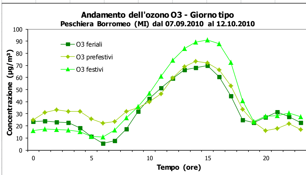
Figura 10: Concentrazioni orarie, medie giornaliere e giorno tipo per O3 a Peschiera Borromeo nel periodo di misura.
