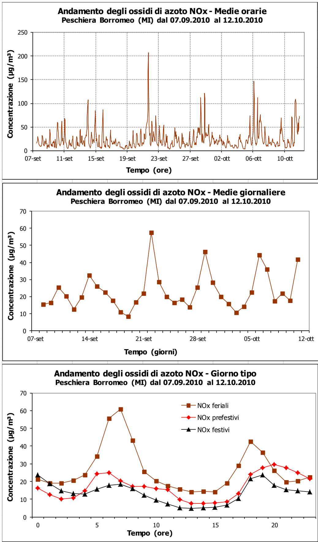
Figura 6: Concentrazioni orarie, medie giornaliere e giorno tipo per NOx a Peschiera Borromeo nel periodo di misura.
