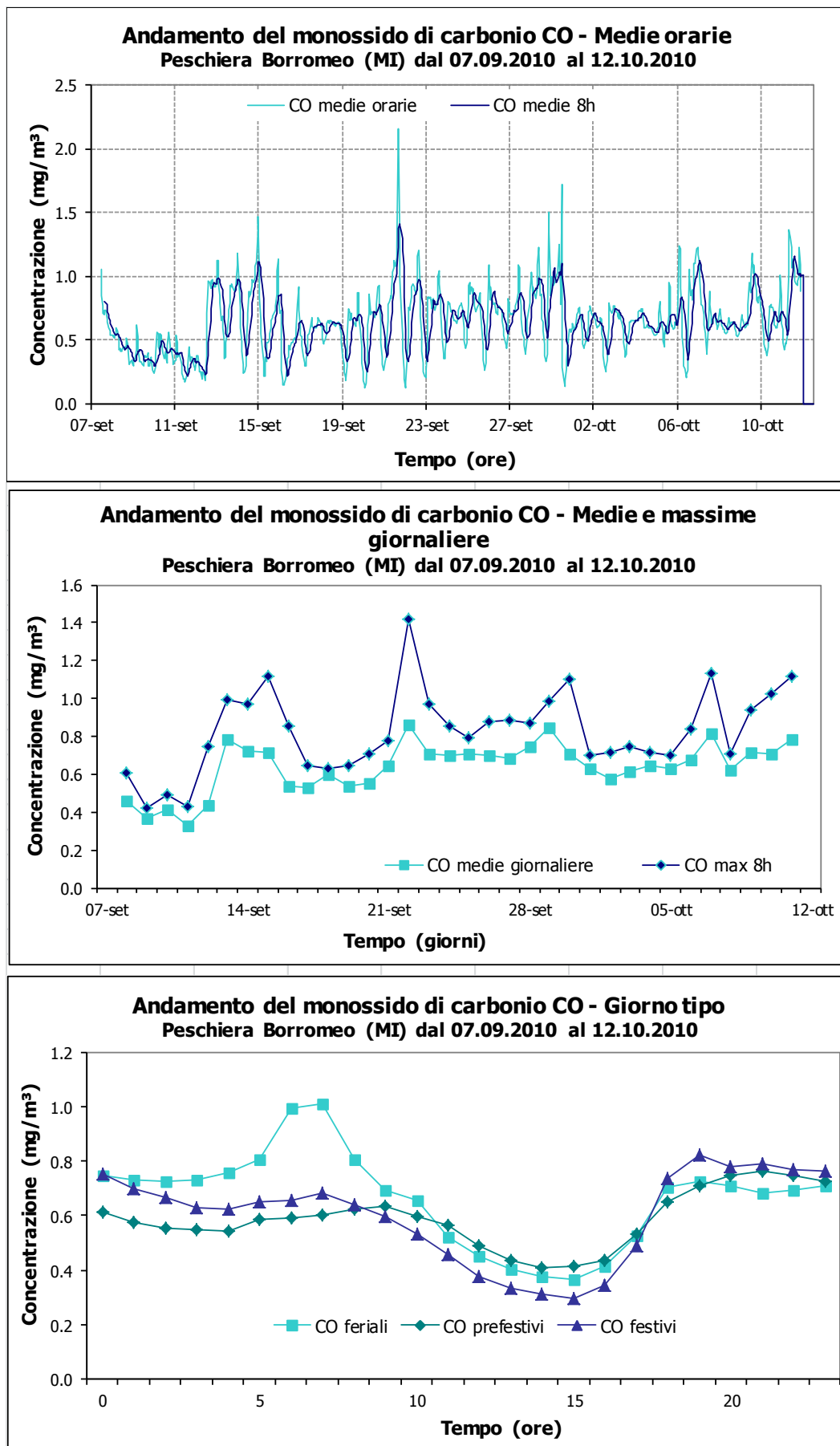
Figura 9: Concentrazioni orarie, medie giornaliere e giorno tipo per CO a Peschiera Borromeo nel periodo di misura.
