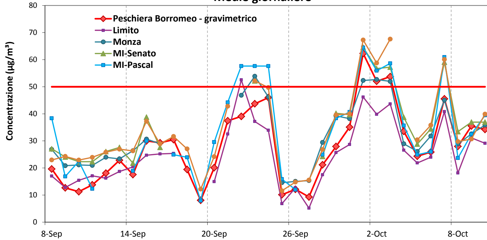
Figura 11: Concentrazioni medie giornaliere di PM10 a Peschiera Borromeo e in alcune stazioni della RRQA nel periodo di misura.
