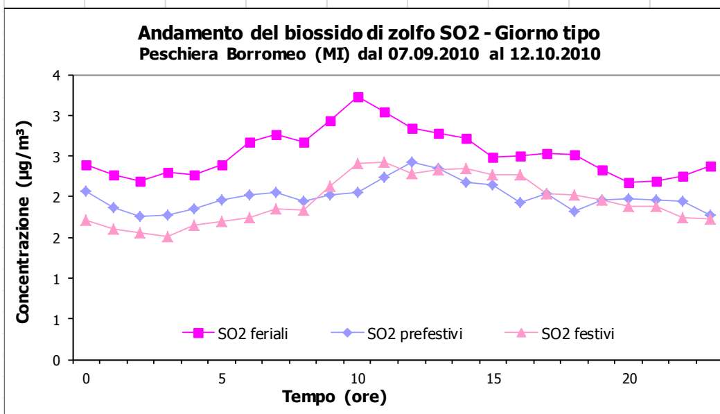
Figura 5: Concentrazioni orarie, medie giornaliere e giorno tipo per SO 2 a Peschiera Borromeo nel periodo di misura.
